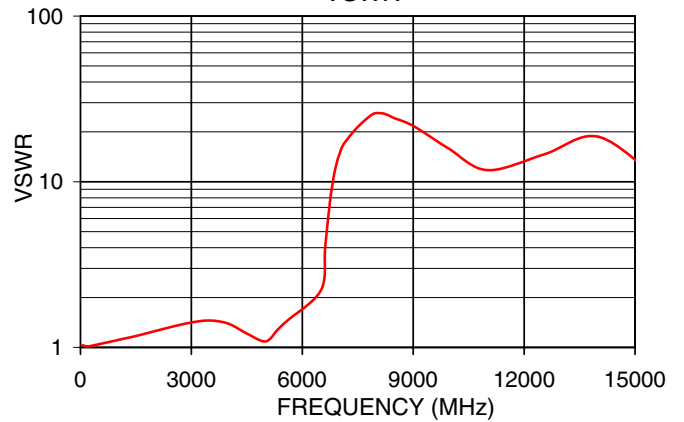
LFCN-5850D+ VSWR
